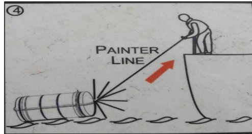
팽창줄을 잡아당긴다.
